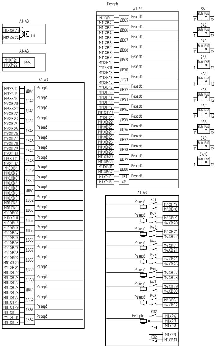
Рисунок Г.9 – Схема электрическая принципиальная (часть 9)
