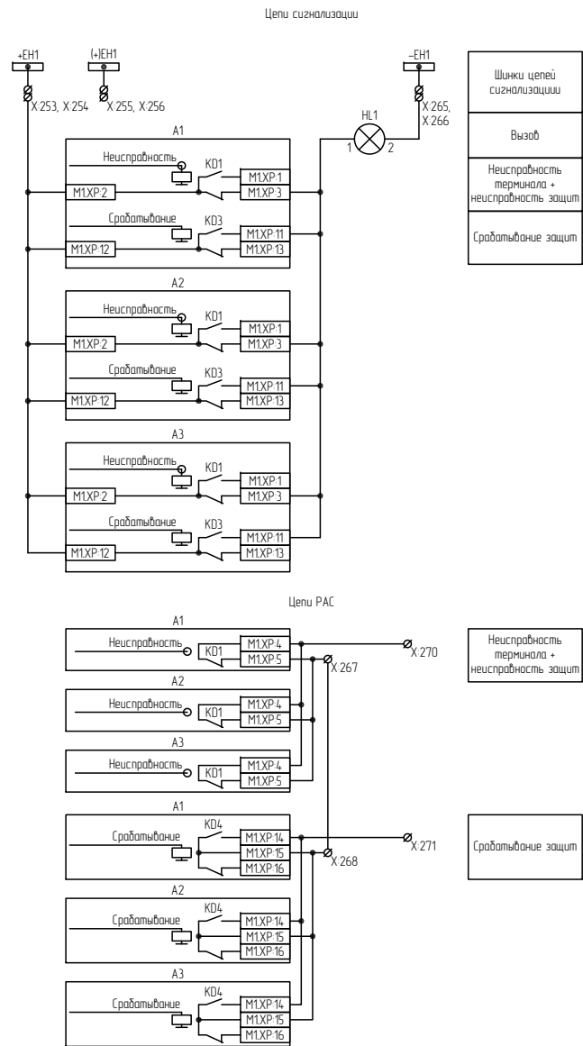
Рисунок Г.8 – Схема электрическая принципиальная (часть 8)
