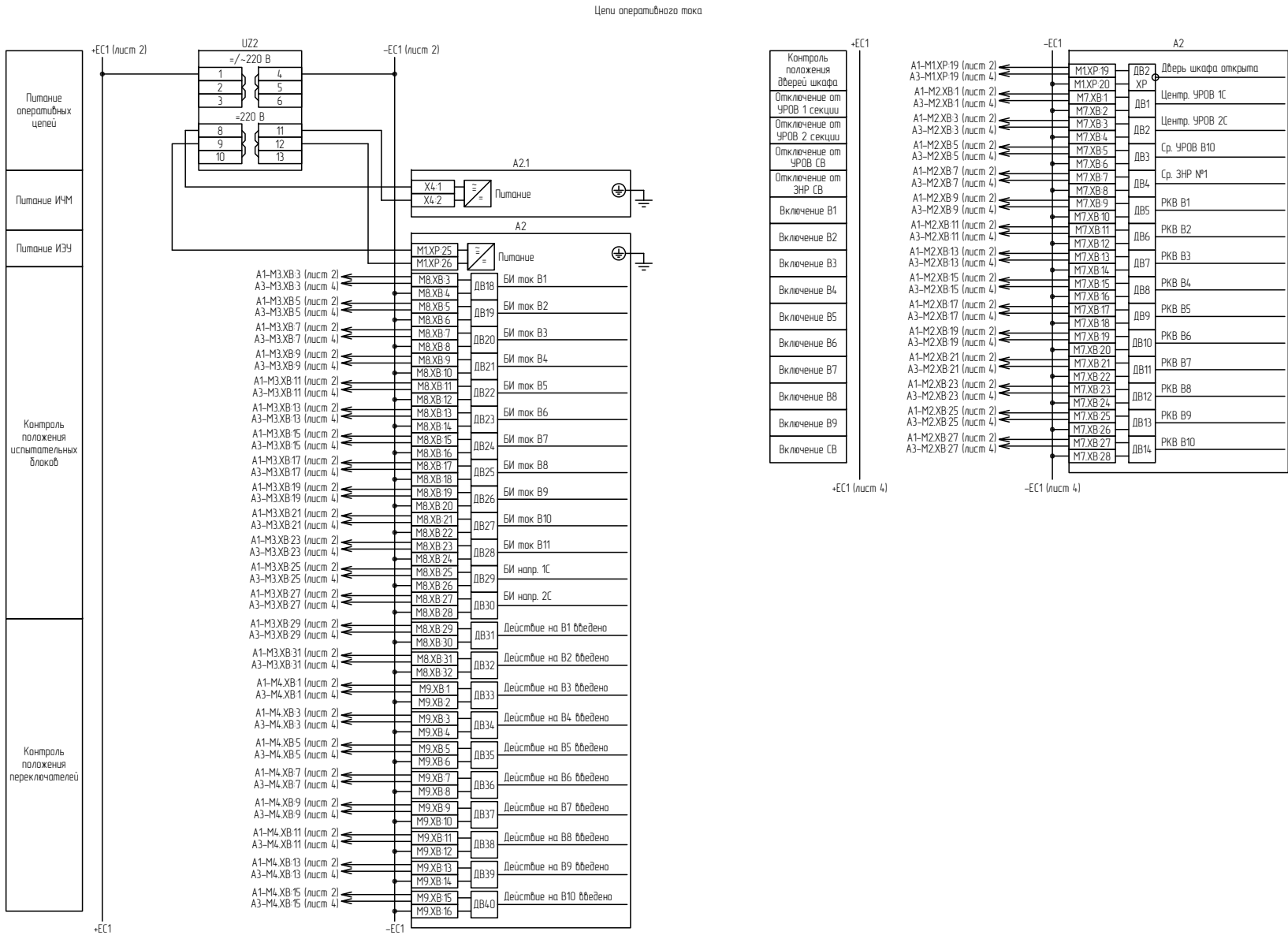
Рисунок Г.3 – Схема электрическая принципиальная (часть 3)
